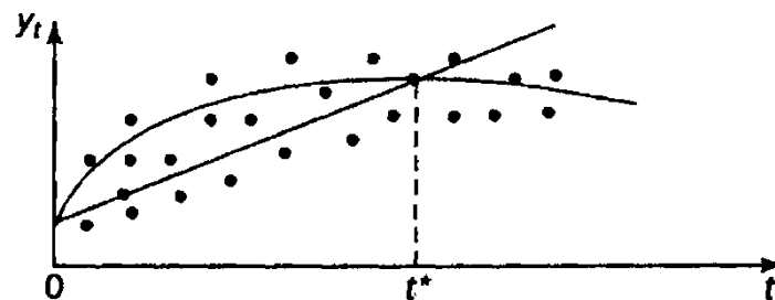
Рис. 4. Ошибка спецификации при выборе уравнения тренда
