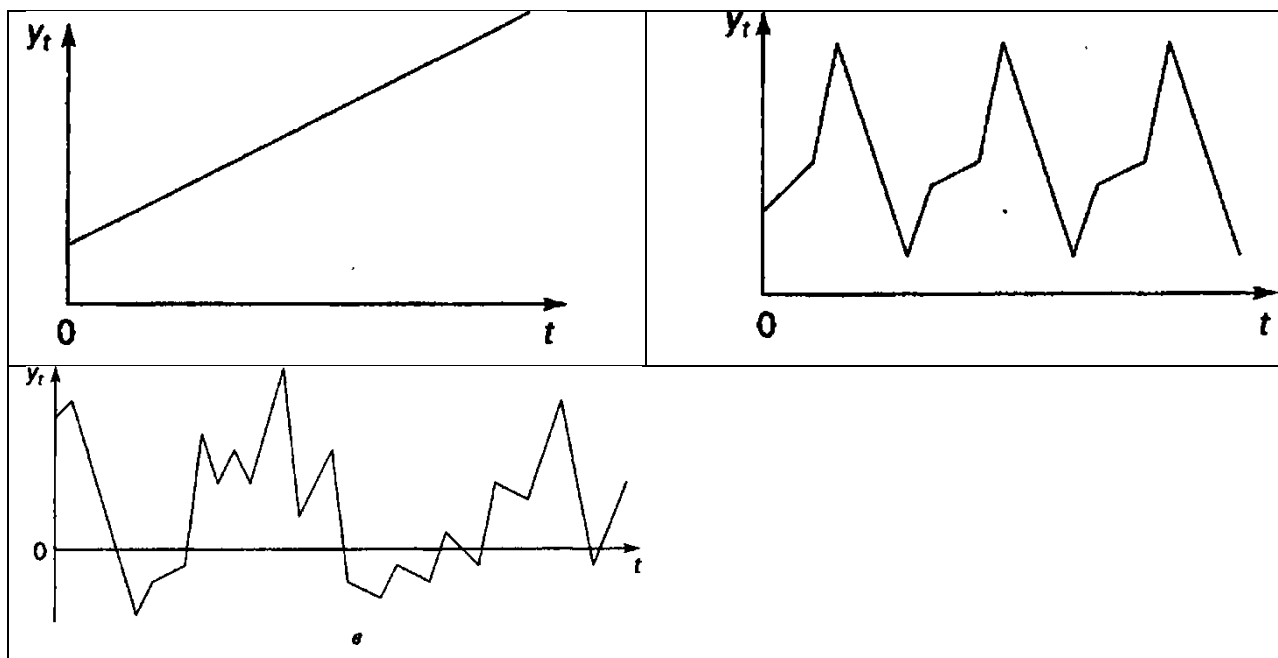
Рис.1. Основные компоненты временного ряда: а - возрастающая тенденция; б - сезонная компонента; в - случайная компонента
